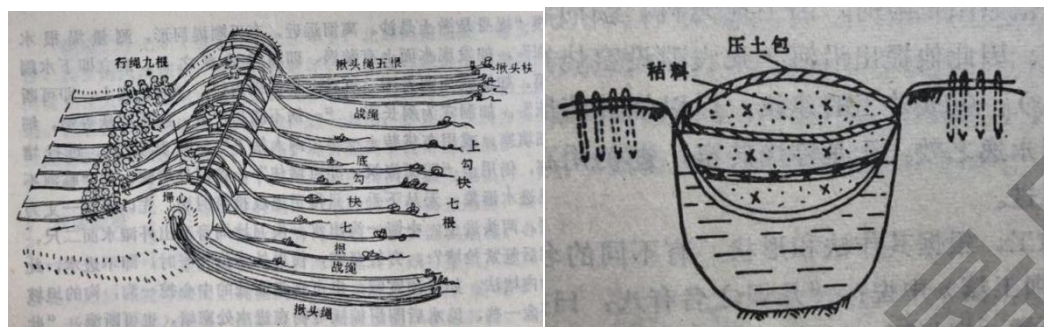
清代卷埽示意图
